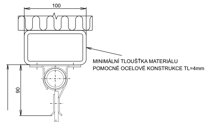
A-A KOTVENÍ DO OCELE
