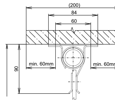
A-A KOTVENÍ DO BETONU
