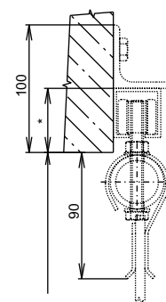
A-A KOTVENÍ DO BETONU
